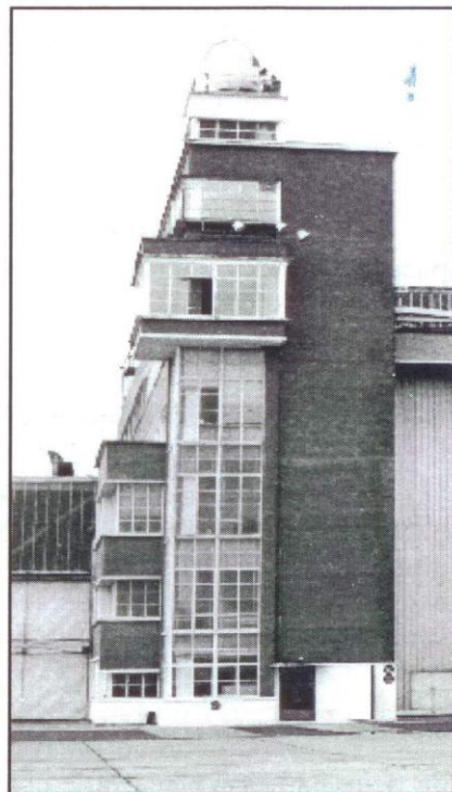
Tour de contrôle équipée d'un cinéthéodolite avec astrodôme et d'un poste de commande.
