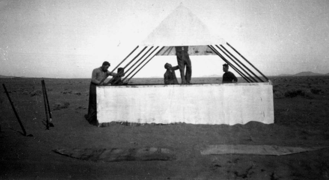
Montage d'une balise. Différents modèles de balises ont été installées de 1929 à 1935, avec des modifications pour améliorer leur visibilité et diminuer leur poids. Ces balises sont placées en bordure des pistes, en principe tous les 10 km (Jean Studer)
